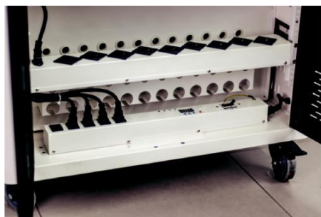
Detail napájacích zásuviek a programovateľného panelu
